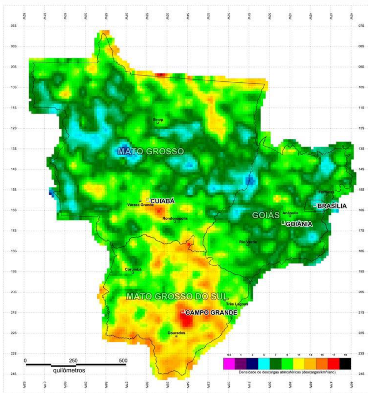
Figura F.4 – Densidade de descargas atmosféricas N_G – Mapa da região centro-oeste (descargas atmosféricas/km²/ano)
